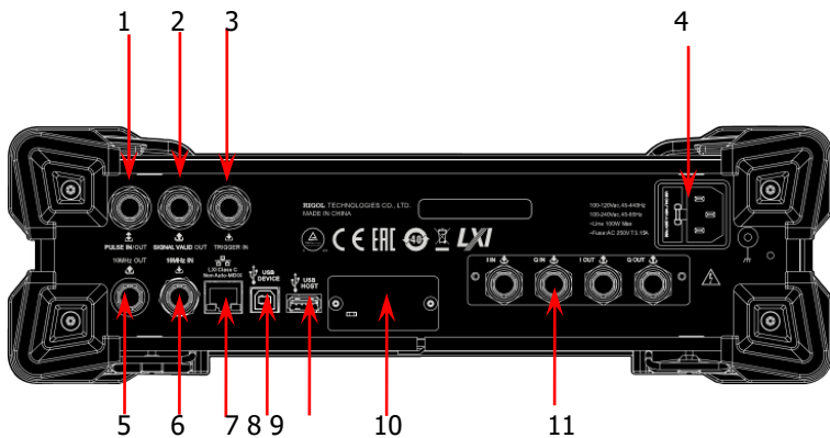
Рисунок 2. Задняя панель
